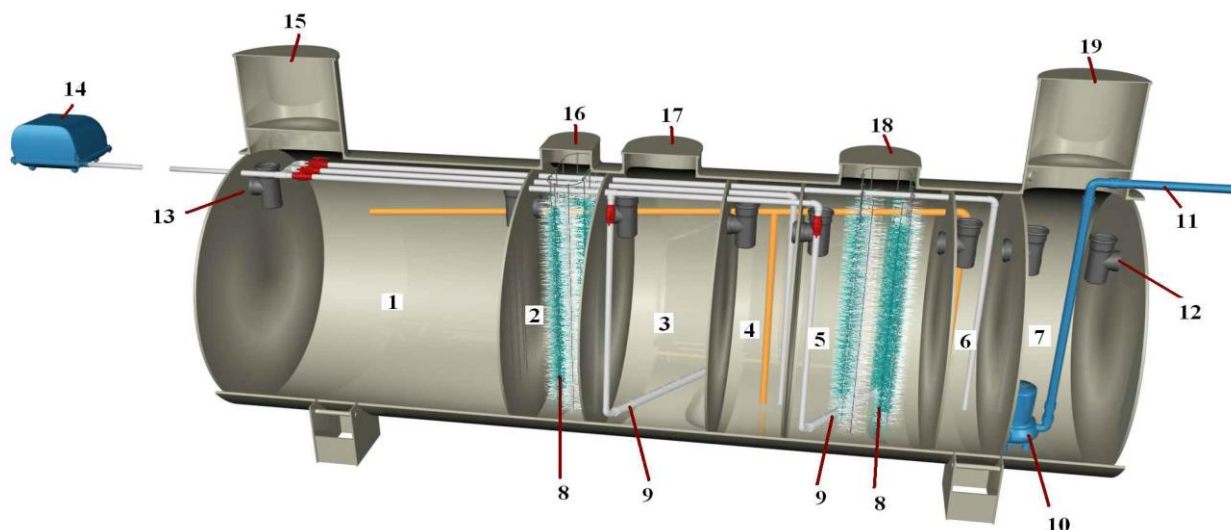
Рис 1. Структурная схема установки 1-Септическая камера-камера минерализации осадка; 2-анаэробной биореактор; 3-аэротенк; 4-вторичный отстойник; 5-биотенк; 6-отсек сбора осадка — третичный отстойник; 7-насосный отсек; 8-ершовая загрузка; 9-аэратор; 10-насос по запросу; 11-трубопровод напорного водоотведения по запросу; 12-трубопровод самотечного водоотведения; 13-вход стоков; 14-компрессор; 15-люк обслуживания септической камеры (конструктив может быть изменен); 16,17,18-
